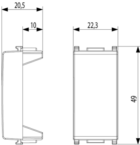
Vista ingombri
