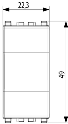
Vista ingombri
