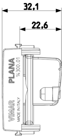
Vista ingombri
